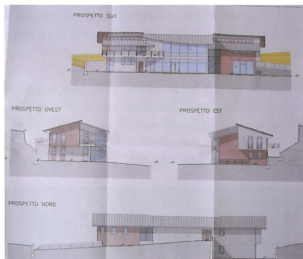
Particolari (prospetti) della nuova casa sociale della frazione di Mala.
