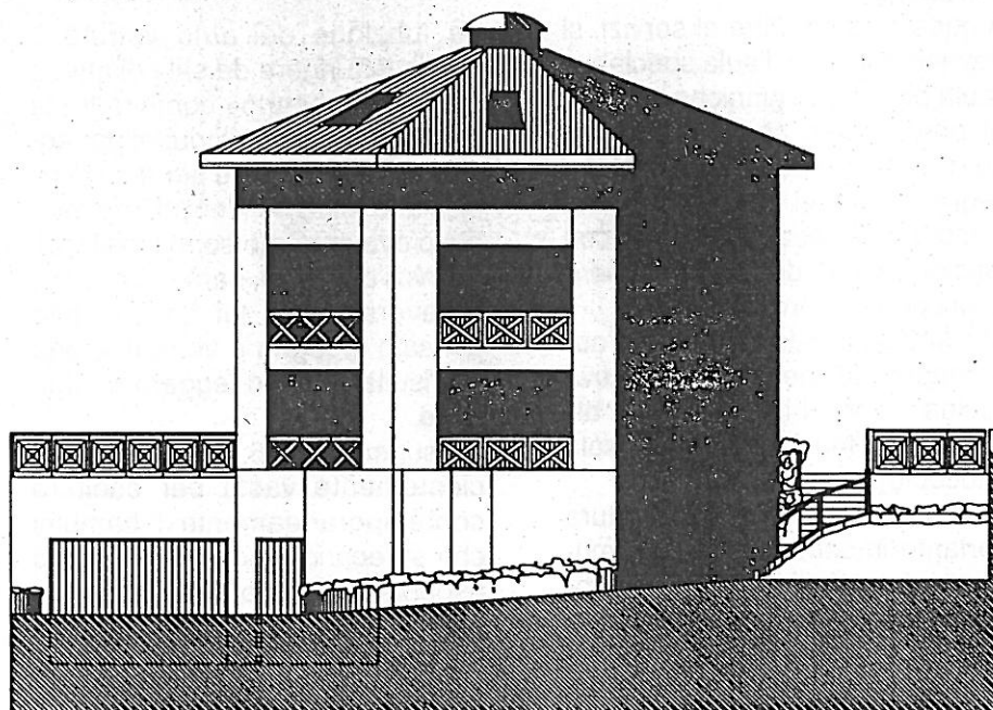
Prospetto dell'edificio polifunzionale.
