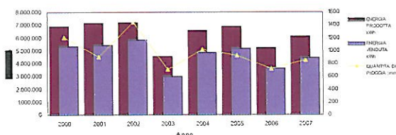
RAPPORTO FRA ENERGIA ELETTRICA PRODOTTA E QUANTITA' DI PIOGGIA
